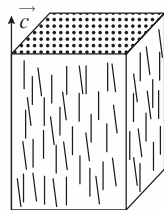
Smectique(A 5 )
