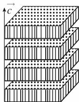
Smectique(A 3 )
