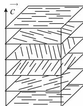
Smectique(A 4 )
